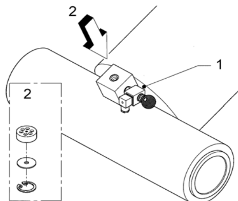
Leiding-/slangbreukbeveiliging
